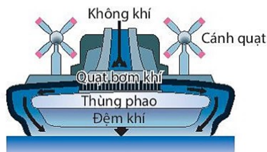
Hình 16.12 Tàu đệm khí
