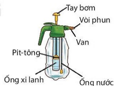
Hình 16.11 Bình xịt nước đơn giản
