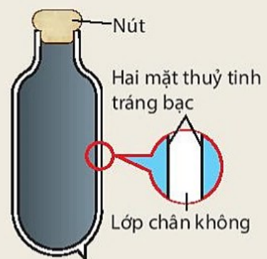
Hình 28.6 Cấu tạo ruột phích (bình thủy)
