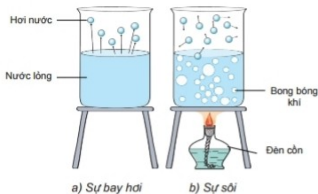
Hình 10.7 Sự bay hơi và sự sôi
