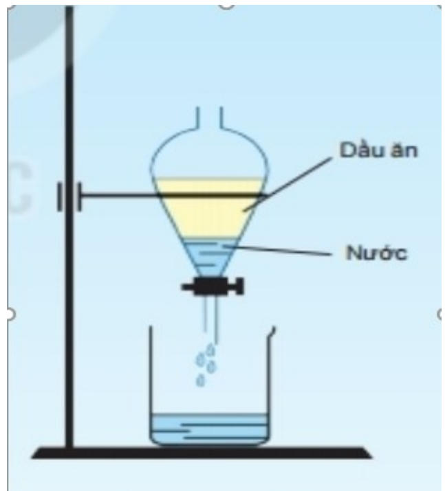
Hình 17.6 Tách dầu ăn khỏi nước bằng phễu chiết
