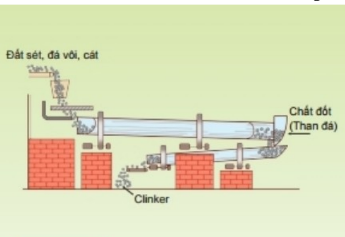
Hình 13.4 Sơ đồ lò quay sản xuất clinker trong quy trình sản xuất xi măng
