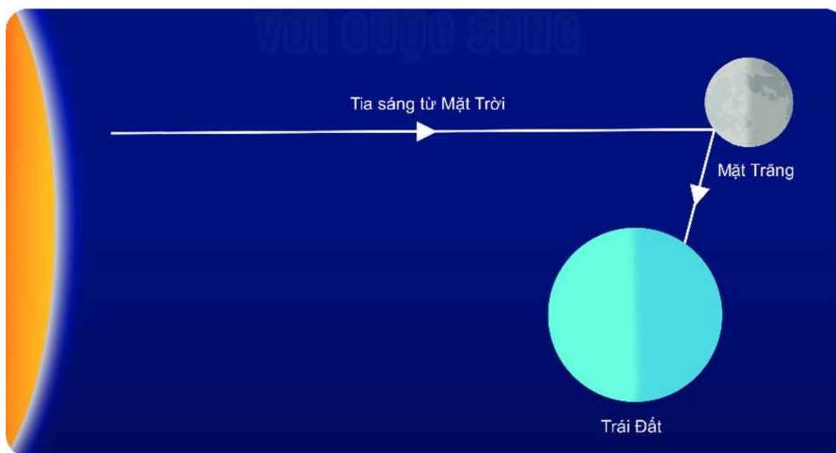
Hình 53.1 Mặt Trời
