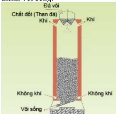
Hình 13.3 Sơ đồ lò nung vôi
