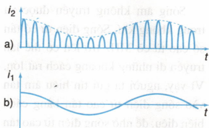
Hình 25.6 Quá trình tách sóng.
