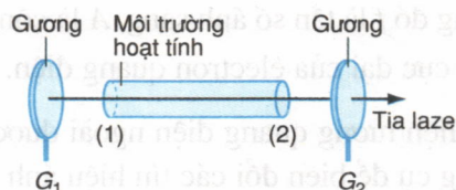
Hình 49.4 Sơ đồ nguyên tắc cấu tạo của laser.
