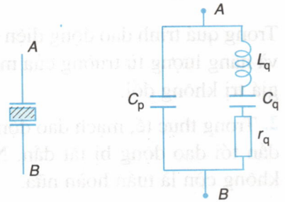
Hình 25.10 Kí hiệu và mạch tương đương của thạch anh.
