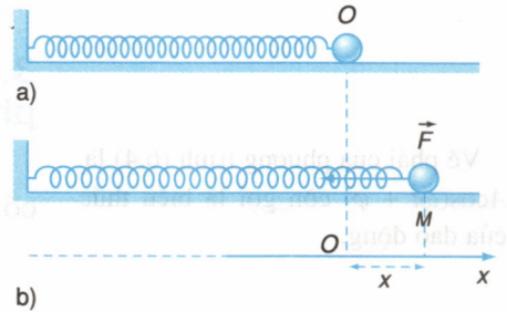
Hình 6.3 Con lắc lò xo.
