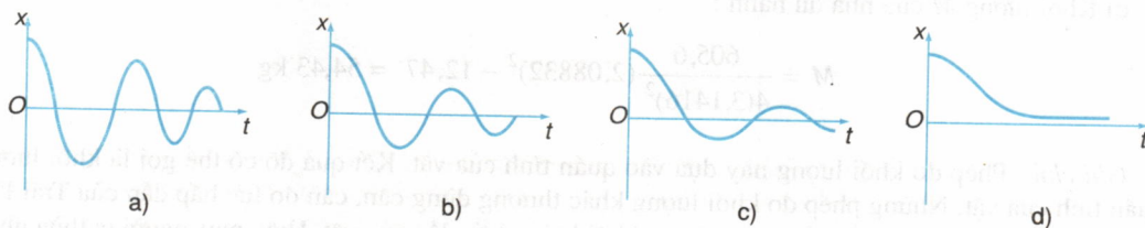
Hình 10.2 Đồ thị của dao động tắt dần.
