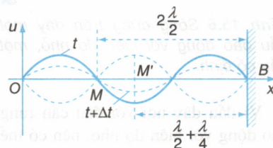
Hình 15.4 Hình dạng sóng dừng ở những thời điểm khác nhau.
