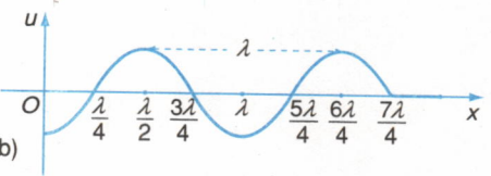
Hình 14.7 Hình dạng thật của sợi dây khi sóng truyền trên sợi dây ở các thời điểm :
