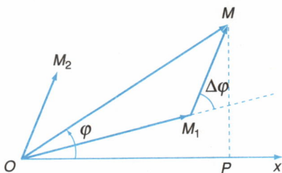
Hình 12.4 Giải đồ Fre-nen để tìm A và φ.
