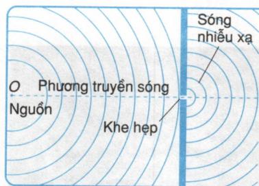
Hình 16.6 Sóng nhiễu xạ qua một khe hẹp.
