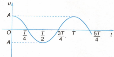
Hình 14.6 Đồ thị biến thiên của li độ u của một phần tử trên đường truyền sóng theo thời gian.
