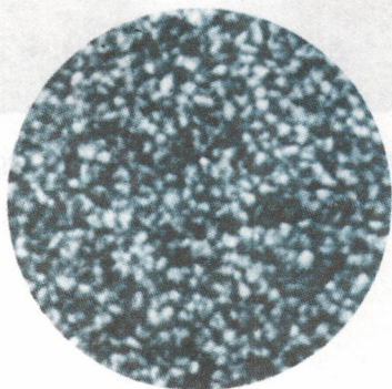
Hình 59.5 Quang cầu.
