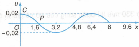
Hình 14.8 Vị trí của phần tử P ở thời điểm t = 3,2 s.
