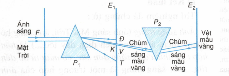
Hình 35.2 Thí nghiệm về ánh sáng đơn sắc.
