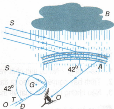
Hình 41.5 Sự tạo thành cầu vồng.
