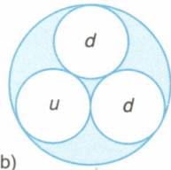
Hình 58.2 Cấu tạo của prôtôn (a) và notron (b).
