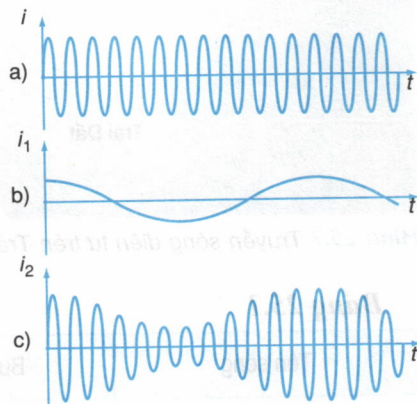
Hình 25.5 Sóng mang (a), tín hiệu âm tần (b) và sóng cao tần biến điệu (c).
