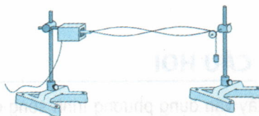
Hình 15.5 Hình dạng sóng dừng trên dây mà mắt nhìn thấy khi f > 24 Hz.
