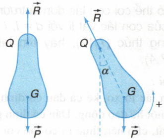
Hình 7.3 Con lắc vật lí.
