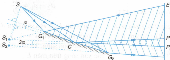
Hình 36.5. Gương Fre-nen.
