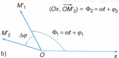
Hình 12.3 Độ lệch pha của hai dao động.
