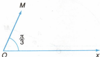
Hình 6.8 Vector quay biểu diễn dao động x .
