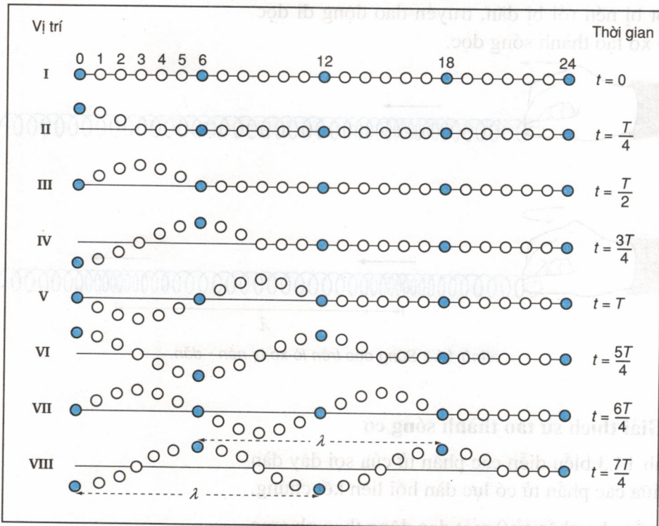
Hình 14.3 Mô hình biểu diễn vị trí của các phần tử của sóng ngang ở những thời điểm liên tiếp.
