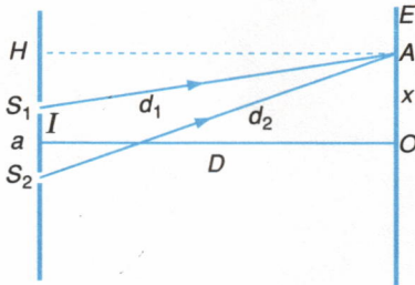
Hình 37.1 Xác định vị trí vân giao thoa.
