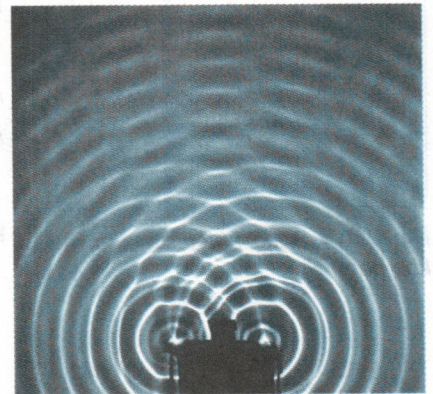
Hình 16.4 Ảnh chụp mặt nước nhìn từ trên xuống khi có giao thoa của hai sóng.
