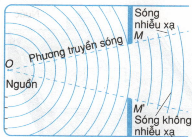
Hình 16.5 Sóng nhiễu xạ qua một khe rộng.
