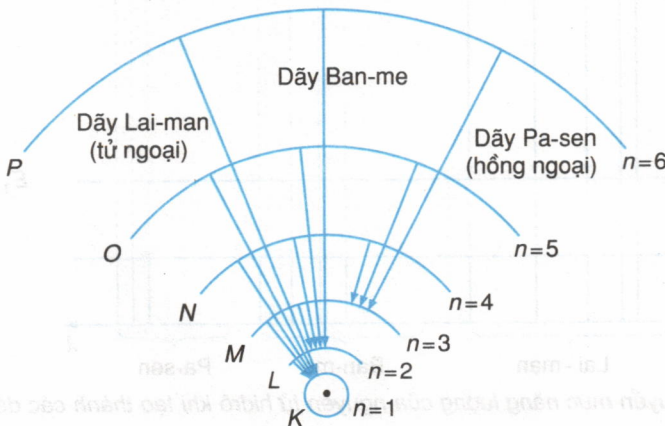
Hình 47.3 Sơ đồ chuyển êlectron từ quỹ đạo này sang quỹ đạo khác khi tạo thành các dãy quang phổ của hiđrô (vẽ phóng chừng độ dài các bán kính).
