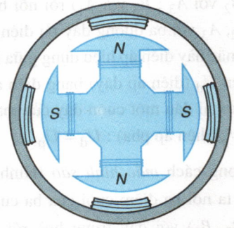
Hình 30.2 Sơ đồ nguyên tắc cấu tạo của một máy phát điện xoay chiều một pha, rôto là nam châm điện có hai cặp cực.
