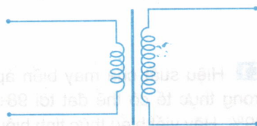
Hình 32.2 Kí hiệu máy biến áp trong mạch điện.
