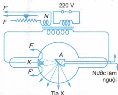
Hình 41.4. Ống Cu-lít-giơ
