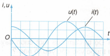
Hình 27.7 Đồ thị biểu diễn sự biến đổi của cường độ dòng điện và điện áp giữa hai đầu cuộn cảm thuần theo thời gian.
