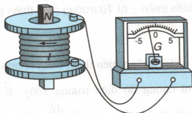
Hình 23.1 Nam châm rơi qua ống dây.
