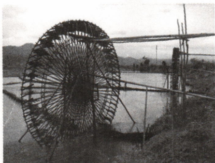
Chuyển động quay của cón nước (loại guồng nước thường thấy ở vùng núi phía Bắc nước ta). Cón nước được dùng để tải nước từ suối lên ruộng cao.
