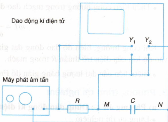
Hình 34.3 Mạch điện khảo sát hai dao động cùng pha.
