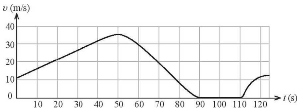
Hình 7.3. Đồ thị vận tốc - thời gian của tàu hỏa
