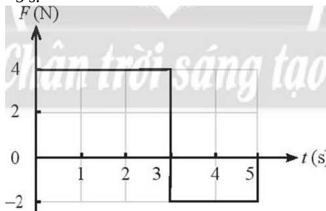
Hình 19.2. Đồ thị lực - thời gian
