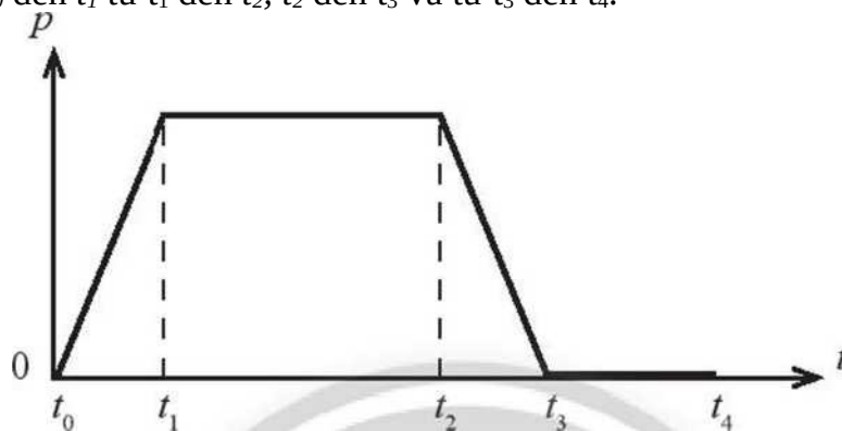
Hình 18.1. Đồ thị động lượng - thời gian
