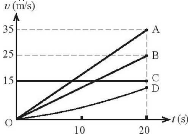
Hình 7.2. Đồ thị vận tốc - thời gian của ô tô A, B, C, D
