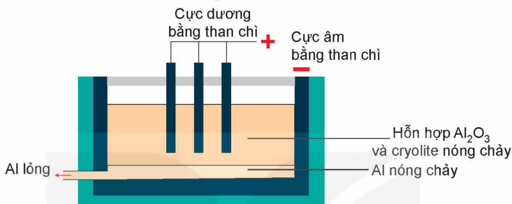
Hình 20.1 Sơ đồ bể điện phân aluminium oxide nóng chảy
