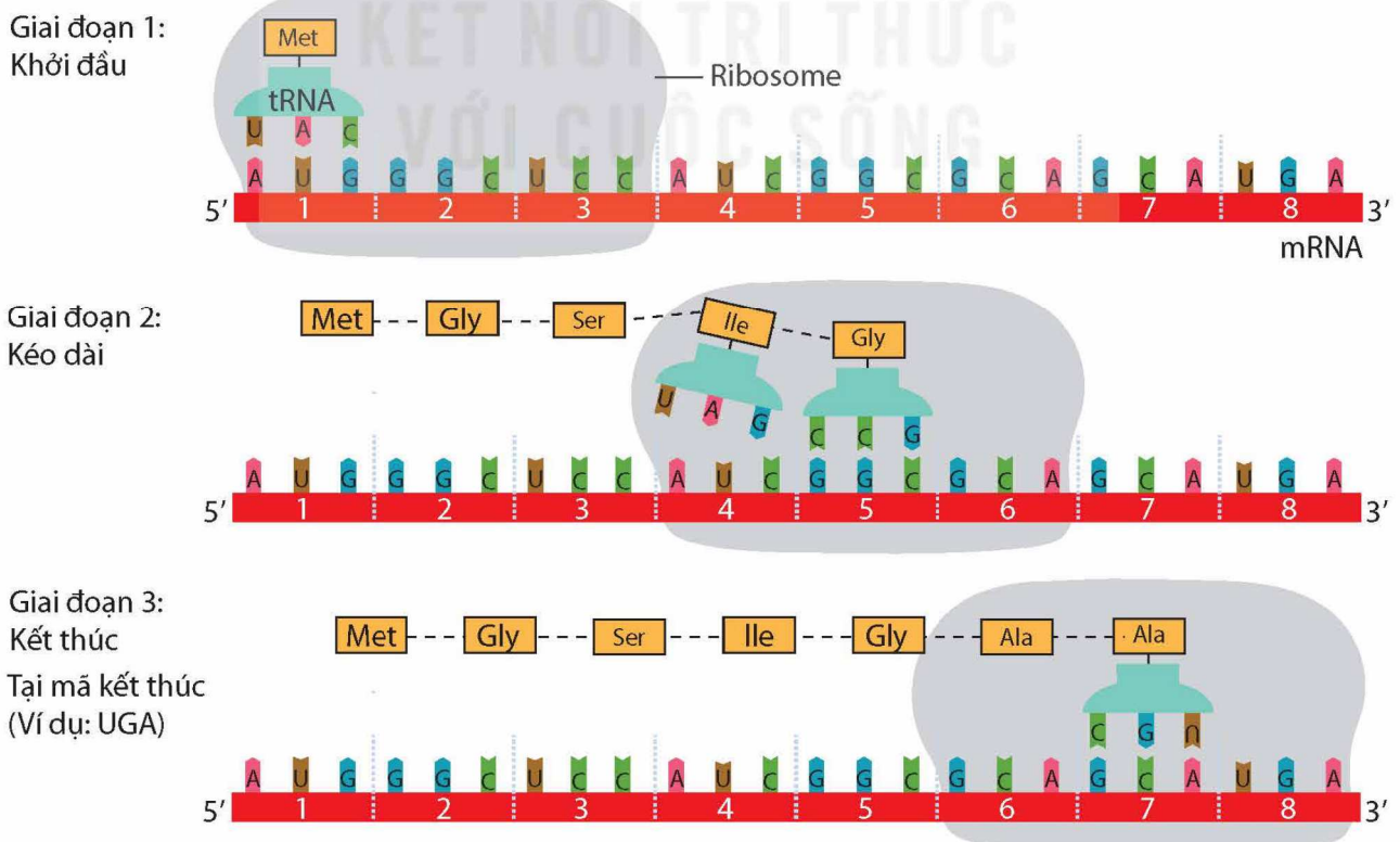
Hình 40.4 Các giai đoạn của quá trình dịch mã
