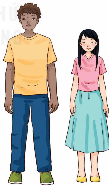
Hình 47.1 Một số tính trạng ở người
