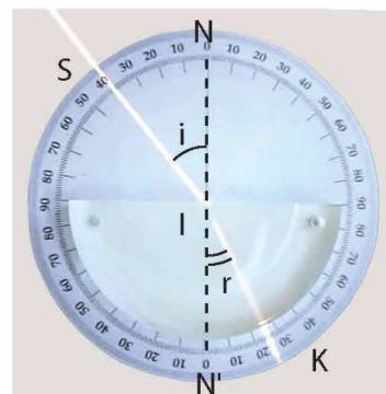
Hình 5.2 Đường truyền của chùm tia sáng
