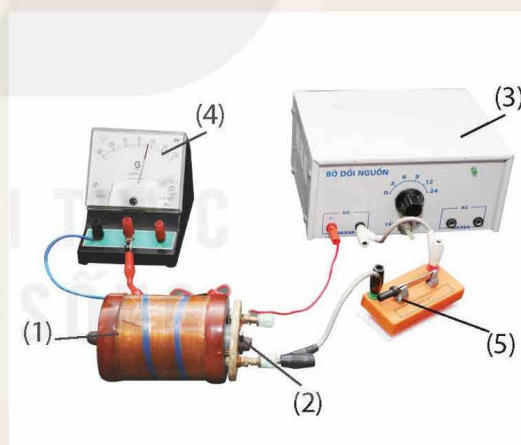
Hình 14.3 Thí nghiệm về dòng điện cảm ứng dùng nam châm điện
