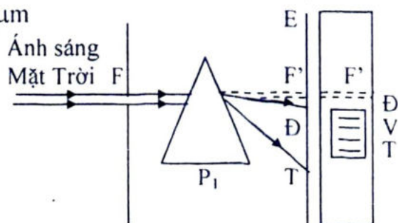
Hình 6.1 Sự tán sắc ánh sáng
