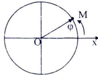
Hình 1.1. Chuyển động tròn của chất điểm
