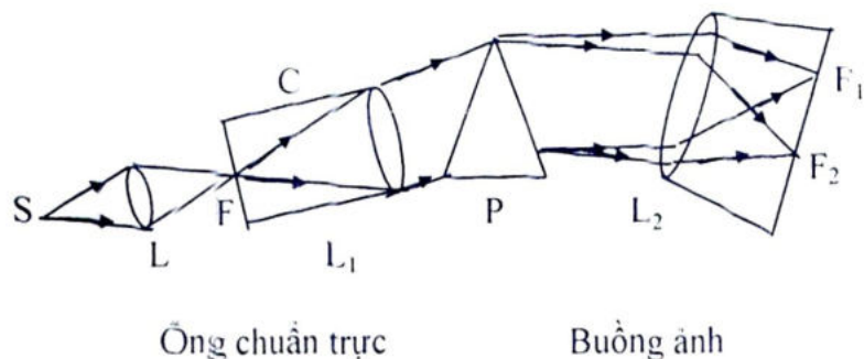
Hình 6.2. Sơ đồ cấu tạo máy quang phổ lăng kính
