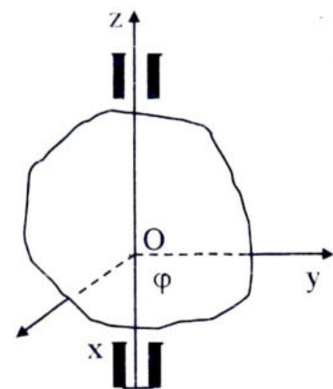
Hình 1.2. Vật rắn với hệ trục tọa độ
