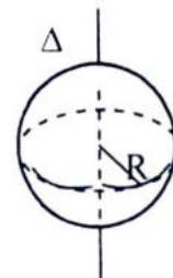
Hình 2.2. Momen quán tính của một số vật đồng chất
