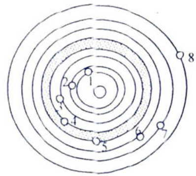
Hình 2.1. Hệ Mặt Trời
