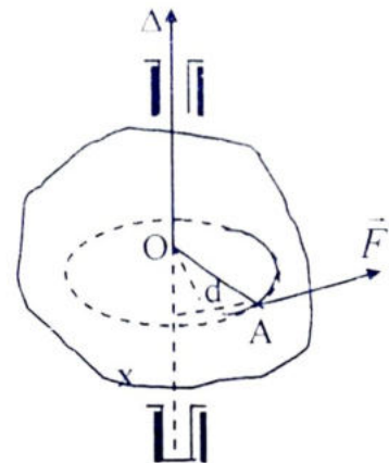
Hình 2.1. Lực \vec{F} và cánh tay đòn d
