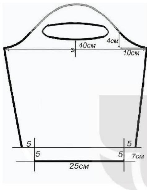
Bản vẽ thông số kích thước
