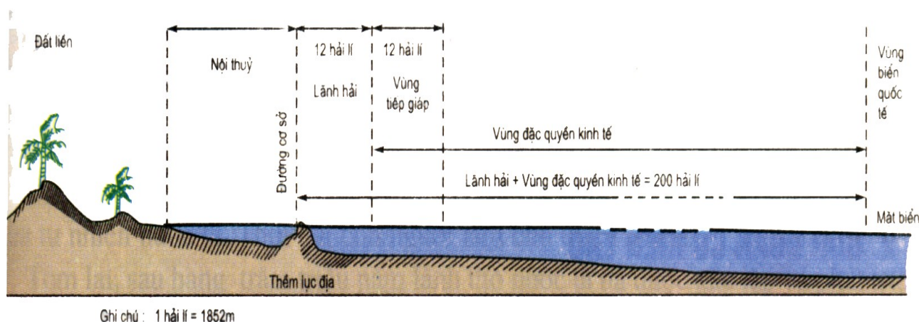
Sơ đồ lát cắt ngang vùng biển Việt Nam
