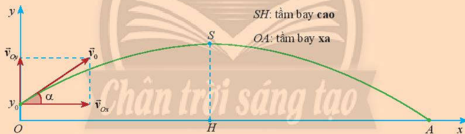
Hình 18. Vật được ném từ vị trí O, với góc ném \alpha bay lên đến điểm cao nhất là S và rơi xuống điểm A
