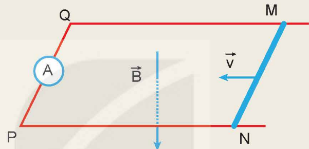
Hình 16.9. Mô tả thí nghiệm thanh kim loại trượt trên hai đoạn dây dẫn
