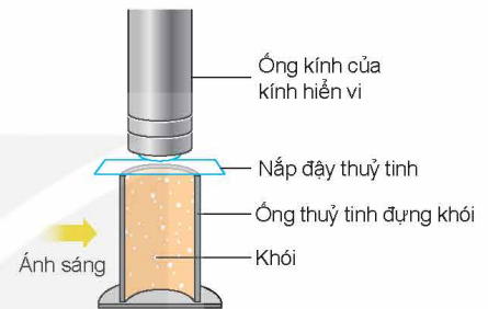
Hình 8.1. Sơ đồ thí nghiệm quan sát chuyển động Brown trong không khí
