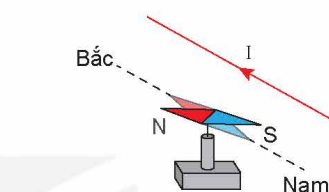
Hình 14.2. Thí nghiệm của Oersted (Ơ-xtét) về tương tác giữa dòng điện và kim nam châm
