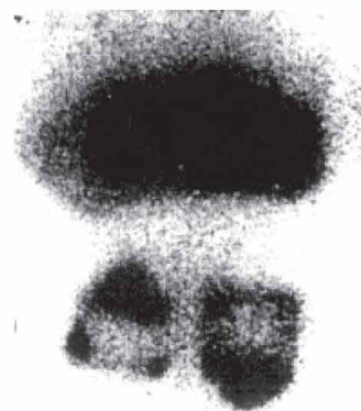
Kết quả thí nghiệm của Becquerel thực hiện năm 1896
