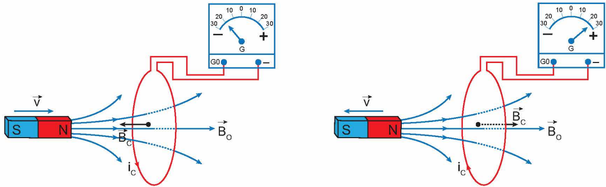
a) Dịch chuyển cực Bắc của nam châm lại gần cuộn dây
