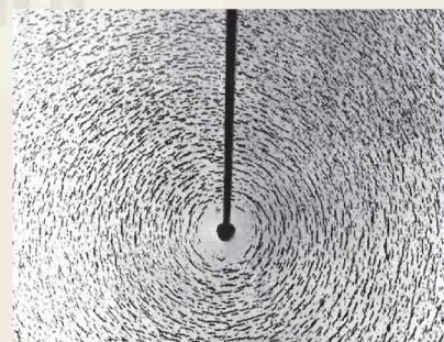
Hình 14.7. Hình ảnh các hạt sắt phân bố xung quanh dòng điện thẳng
