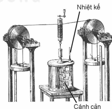
Hình 2.5. Sơ đồ mô tả thí nghiệm của Joule
