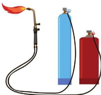
Hình 15.1. Đèn xì acetylene dùng để hàn, cắt kim loại
