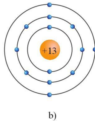
Hình 4.2. Mô hình nguyên tử theo Rutherford – Bohr (a) và cấu trúc nguyên tử aluminium theo mô hình này (b)
