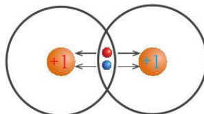
Hình 7.3. Cặp electron liên kết bị các nguyên tử hút về phía các hạt nhân của mỗi nguyên tử H
