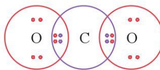
Hình 11.3. Các cặp electron dùng chung và electron hoá trị riêng trong phân tử \text{CO}_2
