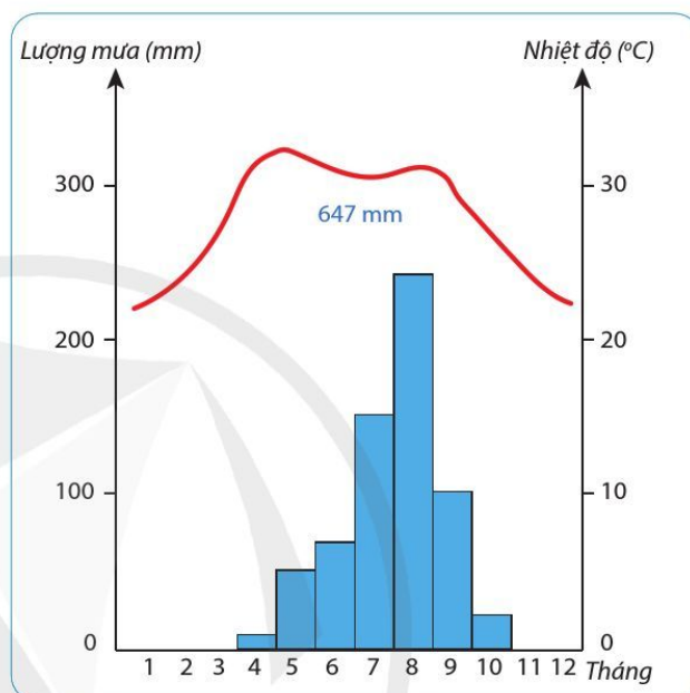
B. Kiểu khí hậu nhiệt đới lục địa (Gia-mê-na, Sát) (12°B, 21°25'Đ)
