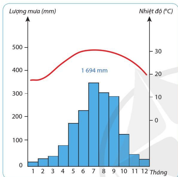
A. Kiểu khí hậu nhiệt đới gió mùa (Hà Nội, Việt Nam) (21°01'B, 105°50'Đ)
