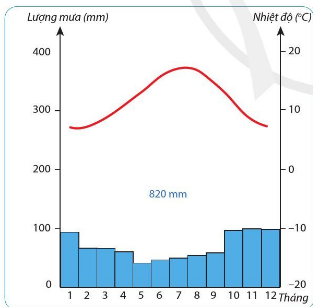
C. Kiểu khí hậu ôn đới hải dương (Bret, Pháp) (48°23'B, 4°29'T)
