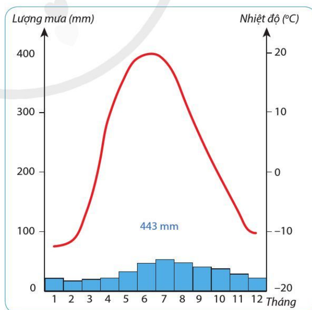
D. Kiểu khí hậu ôn đới lục địa (Ca-dan, Liên bang Nga) (55°47'B, 49°07'Đ)
