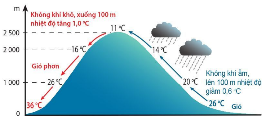
Hình 8.3. Quá trình hình thành gió phơn
