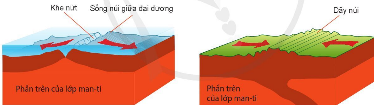
A. Hai mảng kiến tạo tách rời nhau
