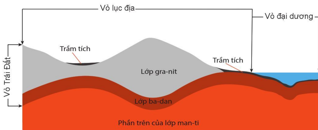
Hình 3.2. Cấu tạo của vỏ Trái Đất
