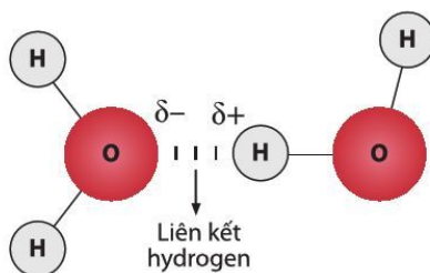
b) Liên kết giữa hai phân tử nước
