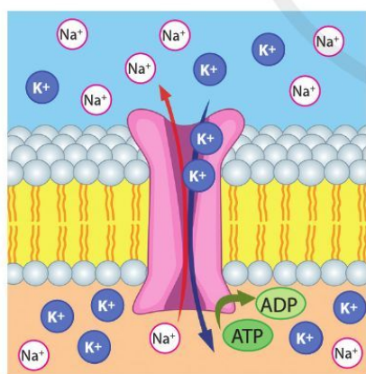
b) Vận chuyển chủ động \text{Na}^+ và \text{K}^+
