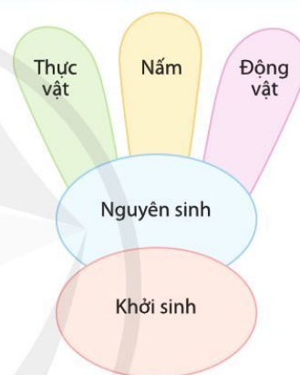
Hình 17.1. Sơ đồ hệ thống phân loại 5 giới sinh vật
