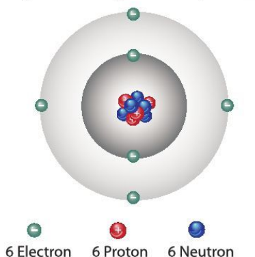
a) Cấu tạo nguyên tử carbon
