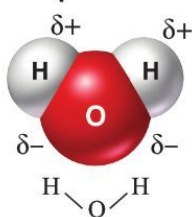
a) Cấu tạo phân tử nước
