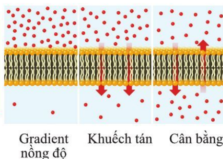
Hình 9.3. Sự khuếch tán qua lớp lipid kép
