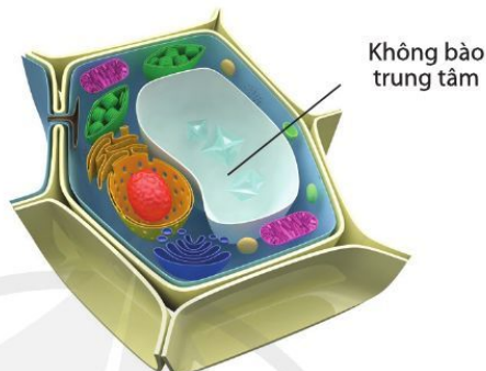
Hình 8.13. Không bào trung tâm ở tế bào thực vật
