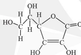
e) Vitamin C
