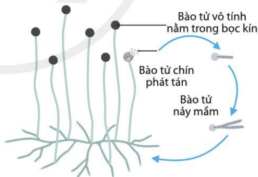
b) Nấm mốc thuộc chi Mucor
