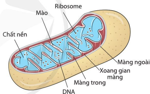
b) Cấu trúc của ti thể
