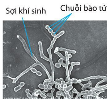
Hình 18.6. Sự hình thành bào tử vô tính ở xạ khuẩn chi Streptomyces (Nguồn: Phùng Thị Ngọc Quyên và Dương Minh Lam)
