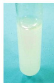
Hình 6.14. Nhũ tương dầu trong nước
