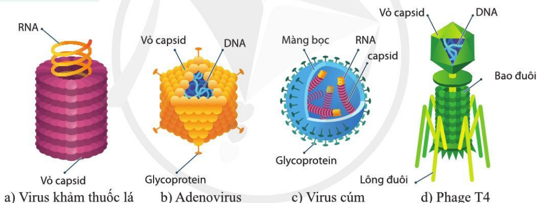
Hình 21.3. Cấu tạo của một số virus
