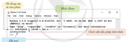
Hình 5. Chương trình tính khoảng cách từ Mặt Trời đến Trái Đất
