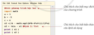
Hình 3. Ghi chú thích trong chương trình
