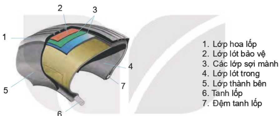
Hình 23.4. Lốp xe ô tô
