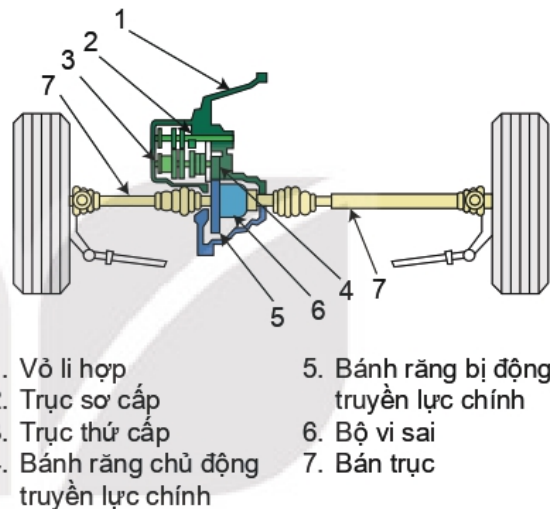
Hình 22.5. Hộp số hai trục gắn liền với bộ truyền lực chính và bộ vi sai
