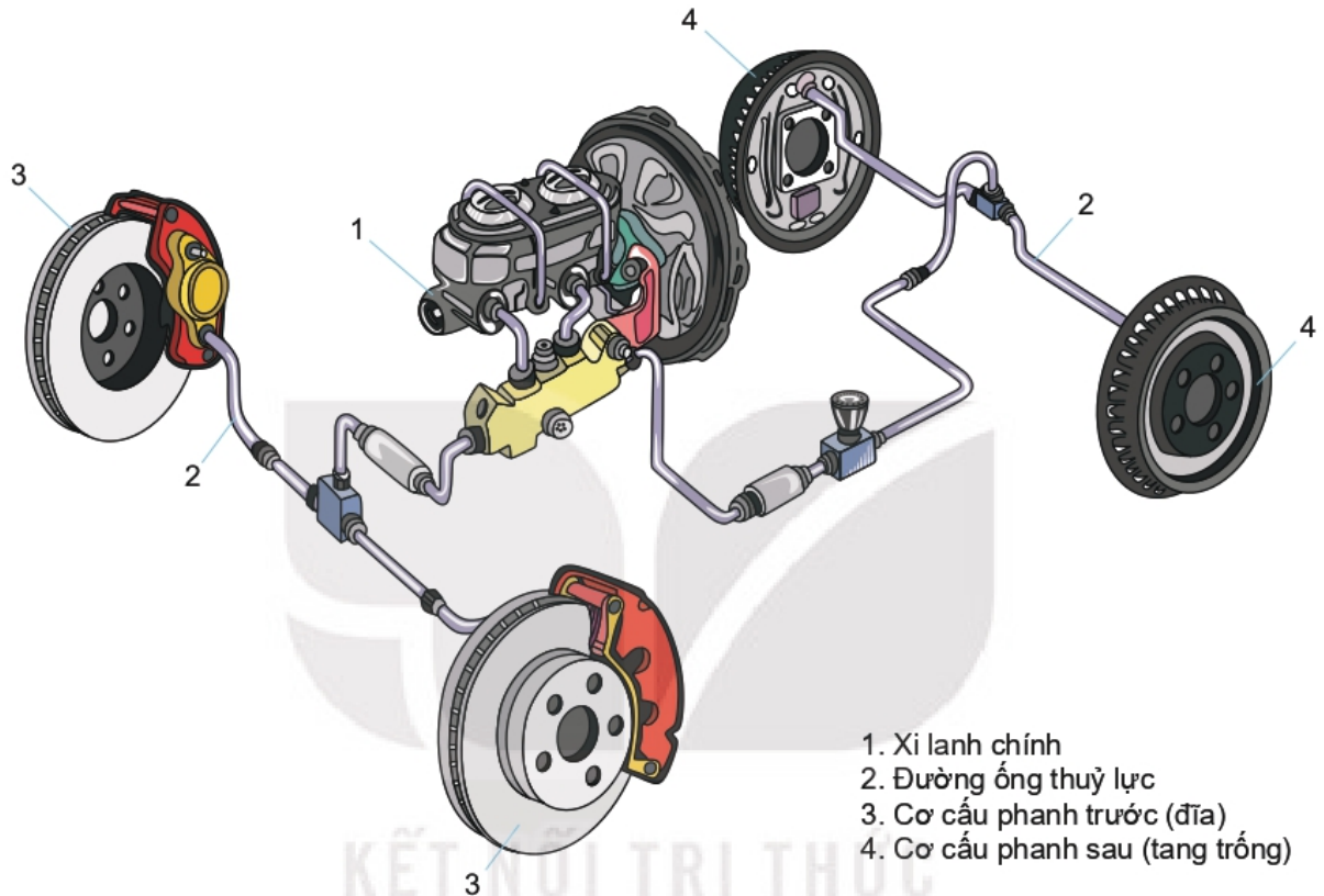
Hình 25.2. Hệ thống phanh trên ô tô con
