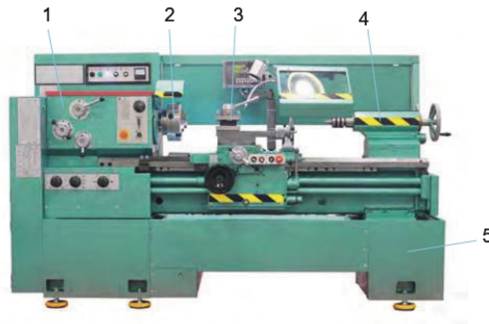
Hình 8.7. Máy tiện vạn năng
