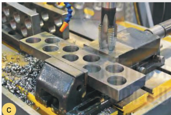
Hình 7.4. Một số phương pháp gia công cơ khí có phoi
