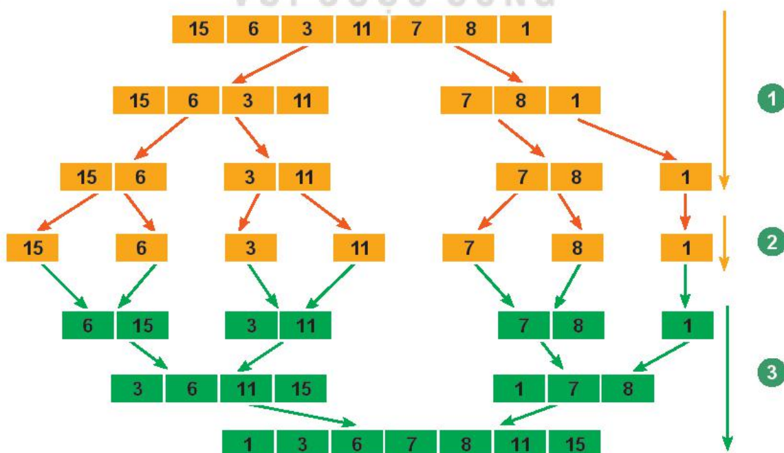
Hình 9.1. Mô phỏng sắp xếp trộn
