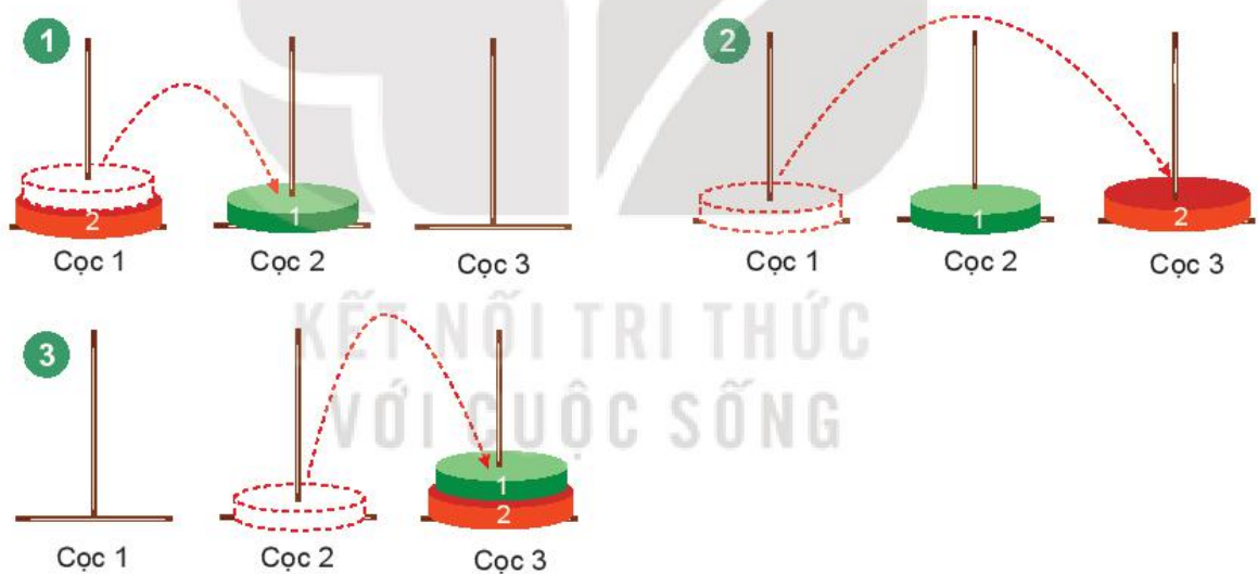
Hình 4.4. Trường hợp n = 2
