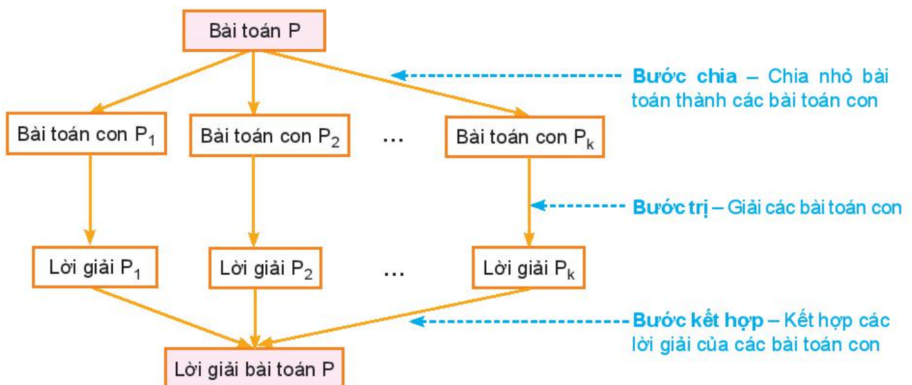
Hình 6.2. Sơ đồ ý tưởng chia để trị
