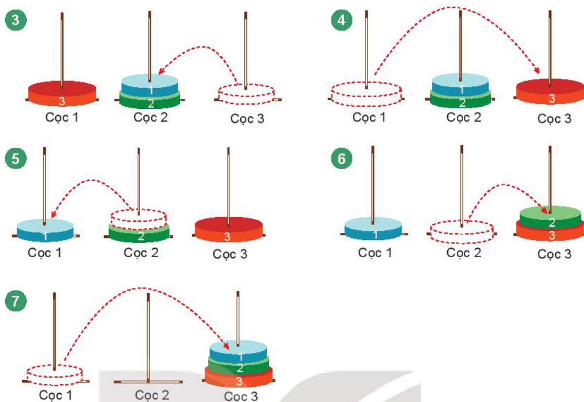
Hình 4.5. Trường hợp n = 3
