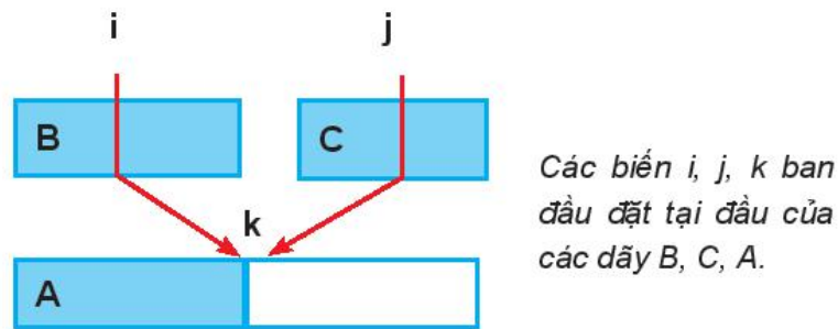
Hình 9.2. Trộn hai dãy B và C
