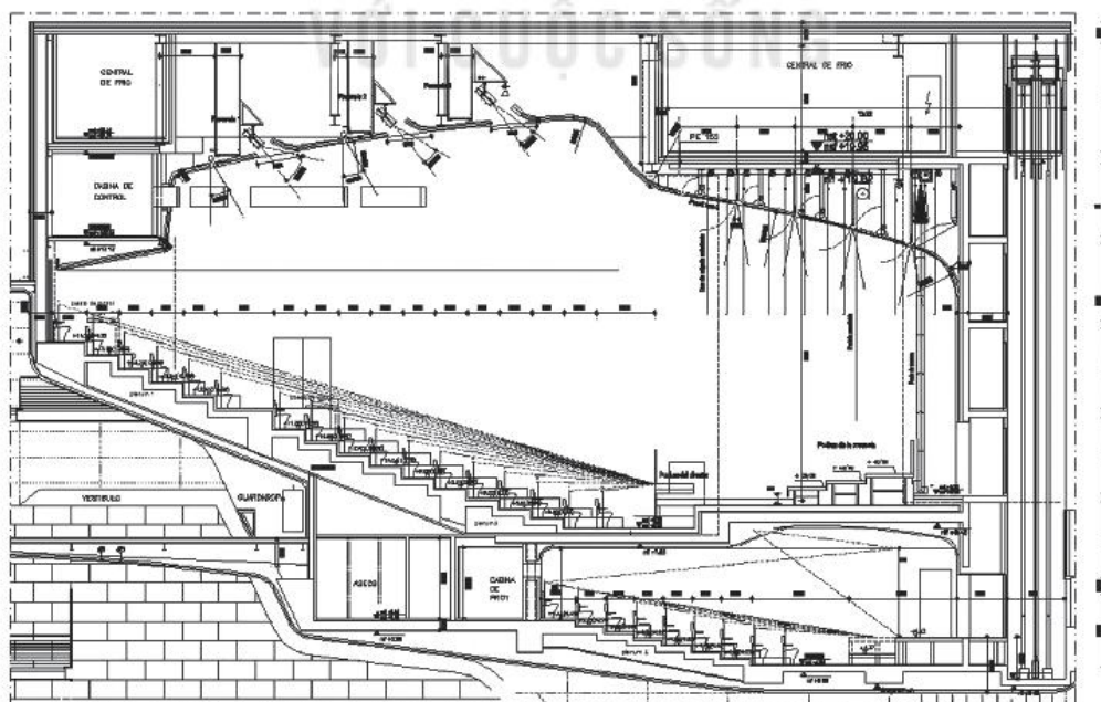
Sơ đồ mặt cắt của một sân khấu (1)
