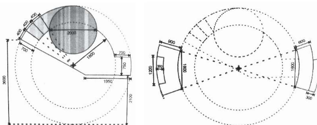
Bản vẽ kĩ thuật khối bục có khung tre (1)
