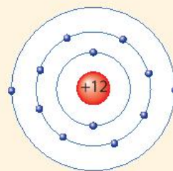
▲ Mô hình nguyên tử magnesium (Mg)
