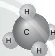
▲ Hình mô phỏng phân tử methane
