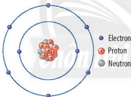
▲ Hình 2.6. Mô hình nguyên tử oxygen (O)
