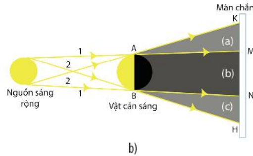
▲ Hình 15.6. a) Thí nghiệm tạo vùng tối bởi một nguồn sáng rộng; b) Hình vẽ biểu diễn vùng tối tạo bởi một nguồn sáng rộng
