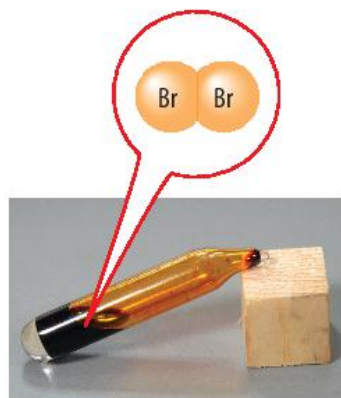
a) Bình chứa bromine lỏng
