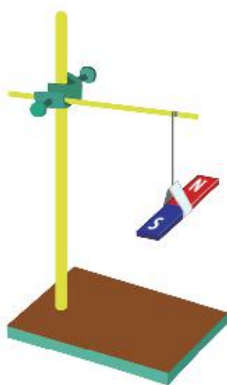
▲ Hình 18.3. Thanh nam châm được treo tự do
