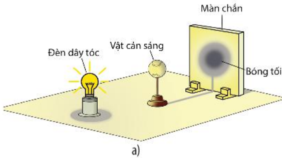
▲ Hình 15.6. a) Thí nghiệm tạo vùng tối bởi một nguồn sáng rộng; b) Hình vẽ biểu diễn vùng tối tạo bởi một nguồn sáng rộng
