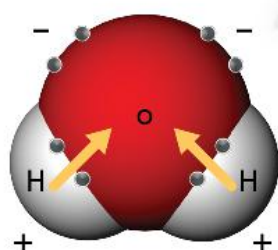
▲ Hình 28.1. Cấu trúc của phân tử nước
