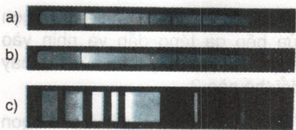
Hình 39.3 Ảnh chụp quang phổ hấp thụ của một số nguyên tố.
