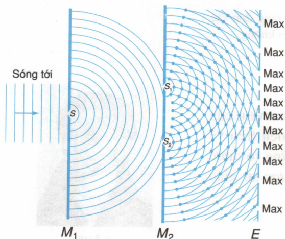
Hình 36.4 Sự giao thoa của hai sóng ánh sáng. Max là vân sáng.
