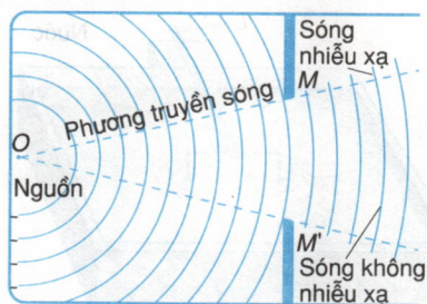
Hình 16.5 Sóng nhiều xạ qua một khe rộng.
