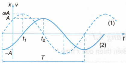
Hình 6.5 Đồ thị vận tốc và đồ thị li độ (pha ban đầu \varphi = 0 ).
