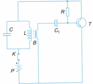
Hình 21.6 Mạch duy trì dao động
