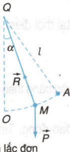
Hình 7.1 Con lắc đơn và sơ đồ.
