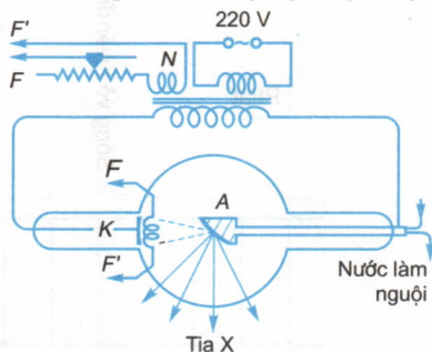
Hình 41.4. Ống Cu-lít-giơ
