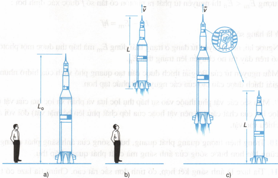
Hình minh họa sự co độ dài của vật theo phương chuyển động.
