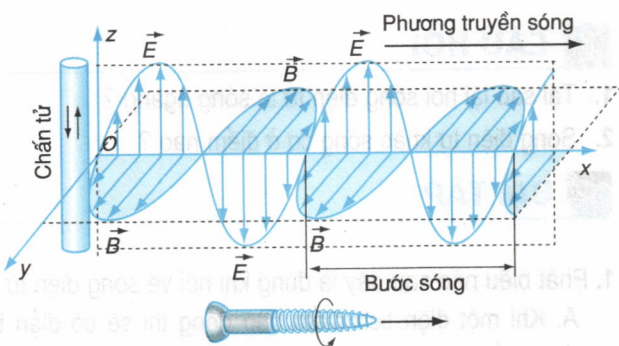
Hình 24.2 Sự lan truyền của sóng điện từ.
