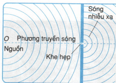
Hình 16.6 Sóng nhiều xạ qua một khe hẹp.
