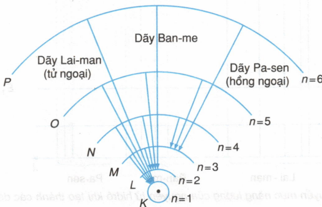
Hình 47.3 Sơ đồ chuyển electron từ quỹ đạo này sang quỹ đạo khác khi tạo thành các dãy quang phổ của hiđrô (vẽ phóng chừng độ dài các bán kính).
