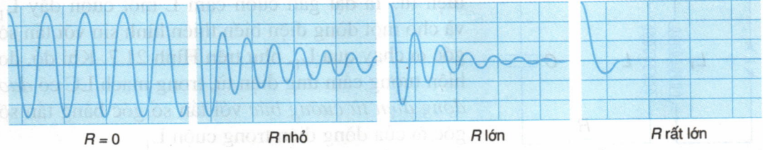
Hình 21.5 Các hình ảnh trên màn hình dao động kí.
