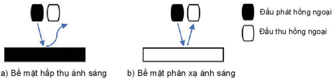
Hình 3.2. Nguyên lý hoạt động của cảm biến dò đường
