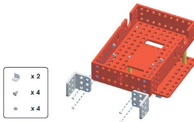
Hình 4.3. Lắp 2 tấm vuông L 2 \times 2 \times 3 vào trước thân 9 \times 15
