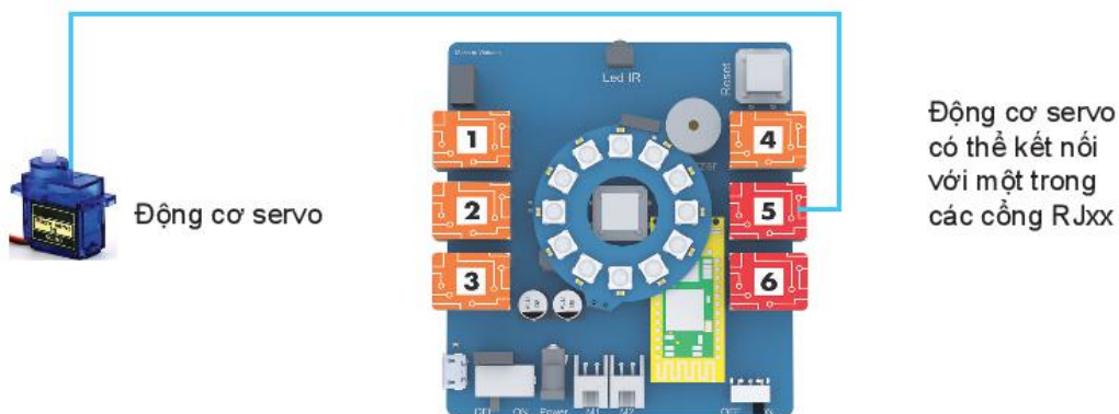
Hình 2.6. Sơ đồ kết nối động cơ servo với robot
