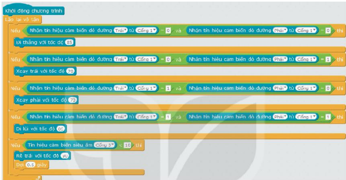
Hình 12.9. Chương trình hoàn thiện để robot thực hiện nhiệm vụ 2
