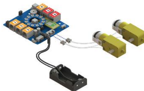
Hình 4.9. Kết nối bảng mạch điều khiển với động cơ M1 và M2
