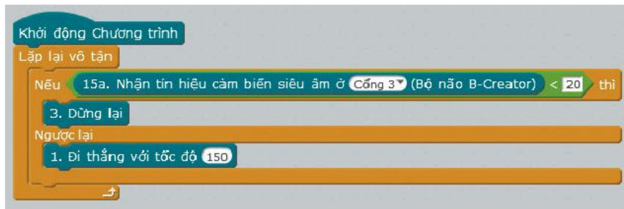
Hình 8.6. Chương trình kiểm tra cảm biến siêu âm
