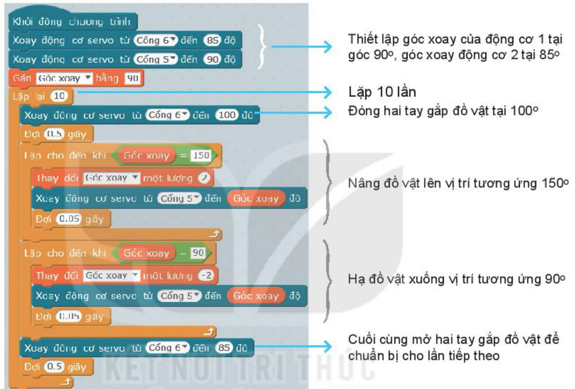
Hình 9.6. Chương trình điều khiển cánh tay hai bậc của robot G-Robot
