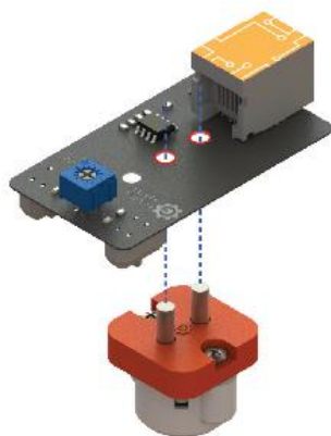
Hình 4.11. Lắp ghép cảm biến dò đường vào bánh xe đa hướng
