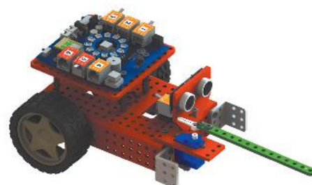
Hình 14.7. Robot sử dụng động cơ servo làm cơ cấu dọn dẹp vật cản
