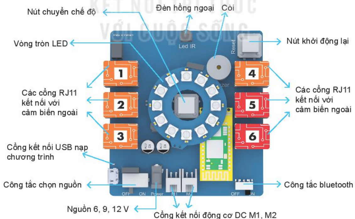
Hình 2.2. Bảng mạch điều khiển của G-Robot
