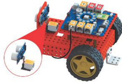
Hình 4.14. Gắn bộ chuyển đổi cảm biến siêu âm vào cảm biến siêu âm
