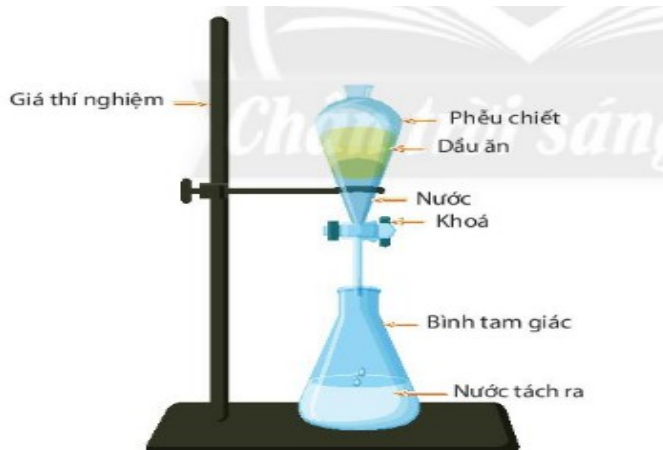
▲ Hình 16.5. Tách chất bằng phễu chiết
