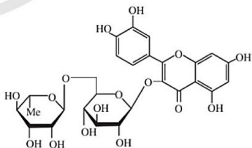
rutin
